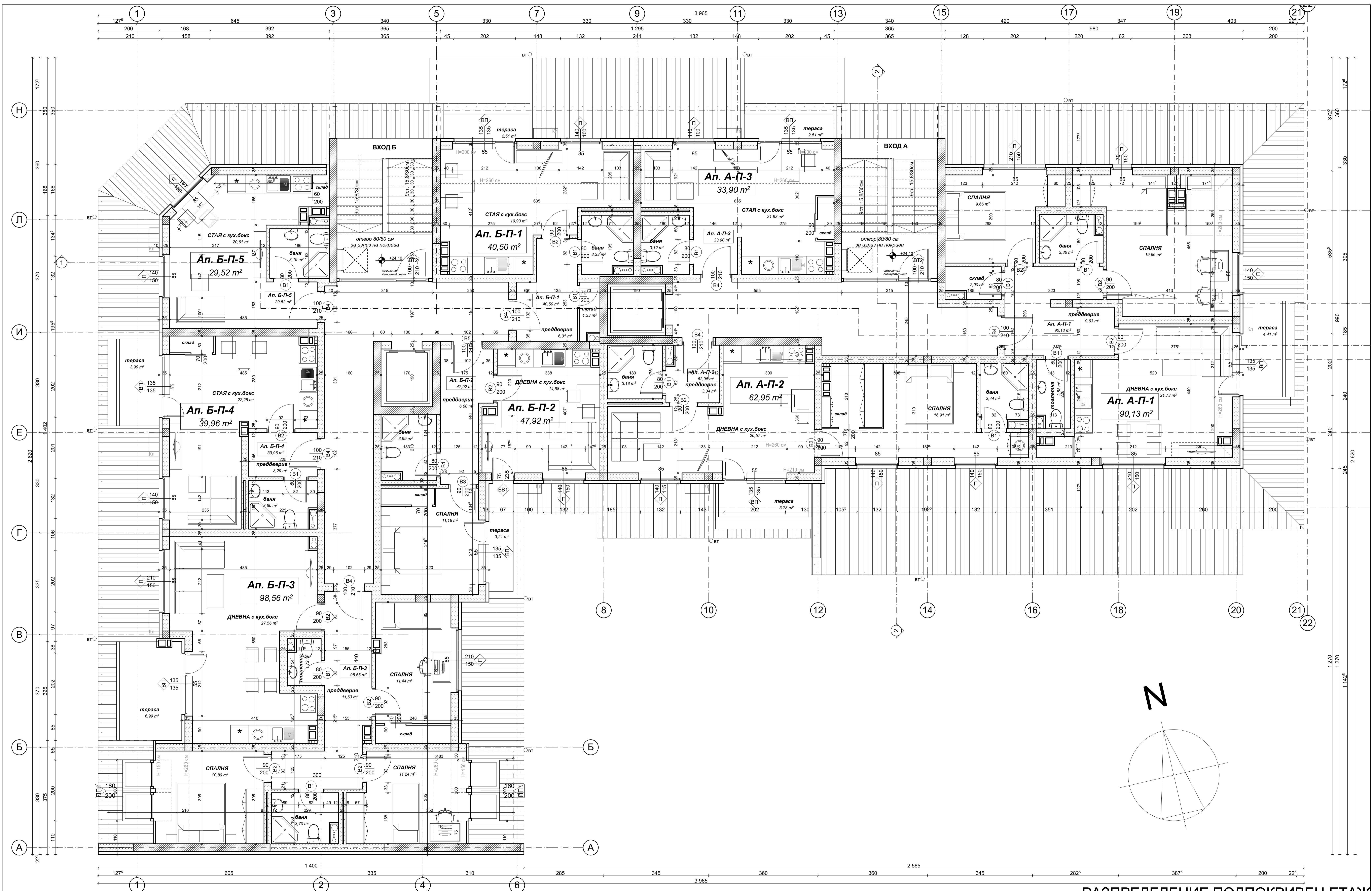
РАЗПРЕДЕЛЕНИЕ ПОДПОКРИВЕН ЕТАЖ
