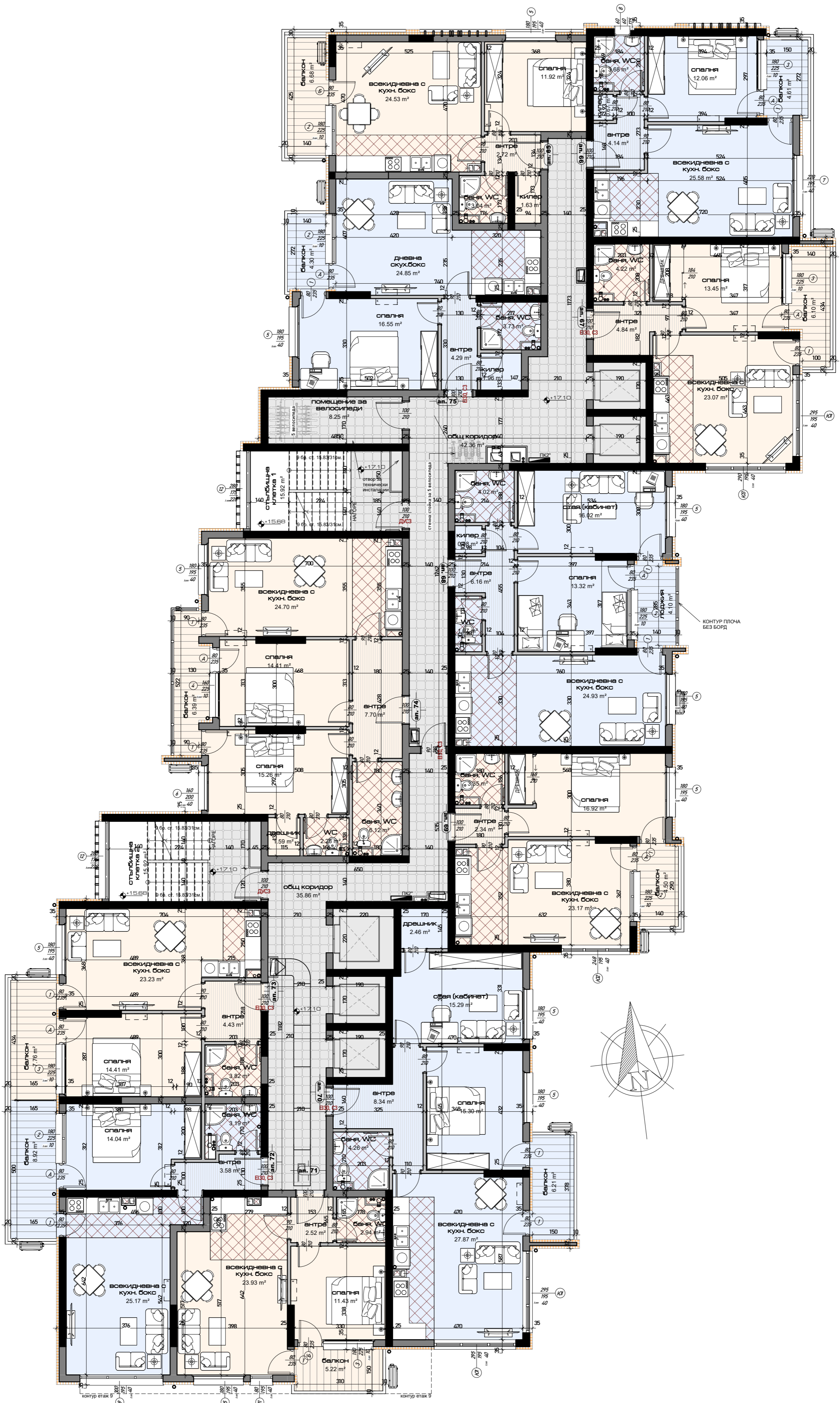
13 РАЗПРЕДЕЛЕНИЕ ЕТАЖ 8 (кт. +17.10м.)
