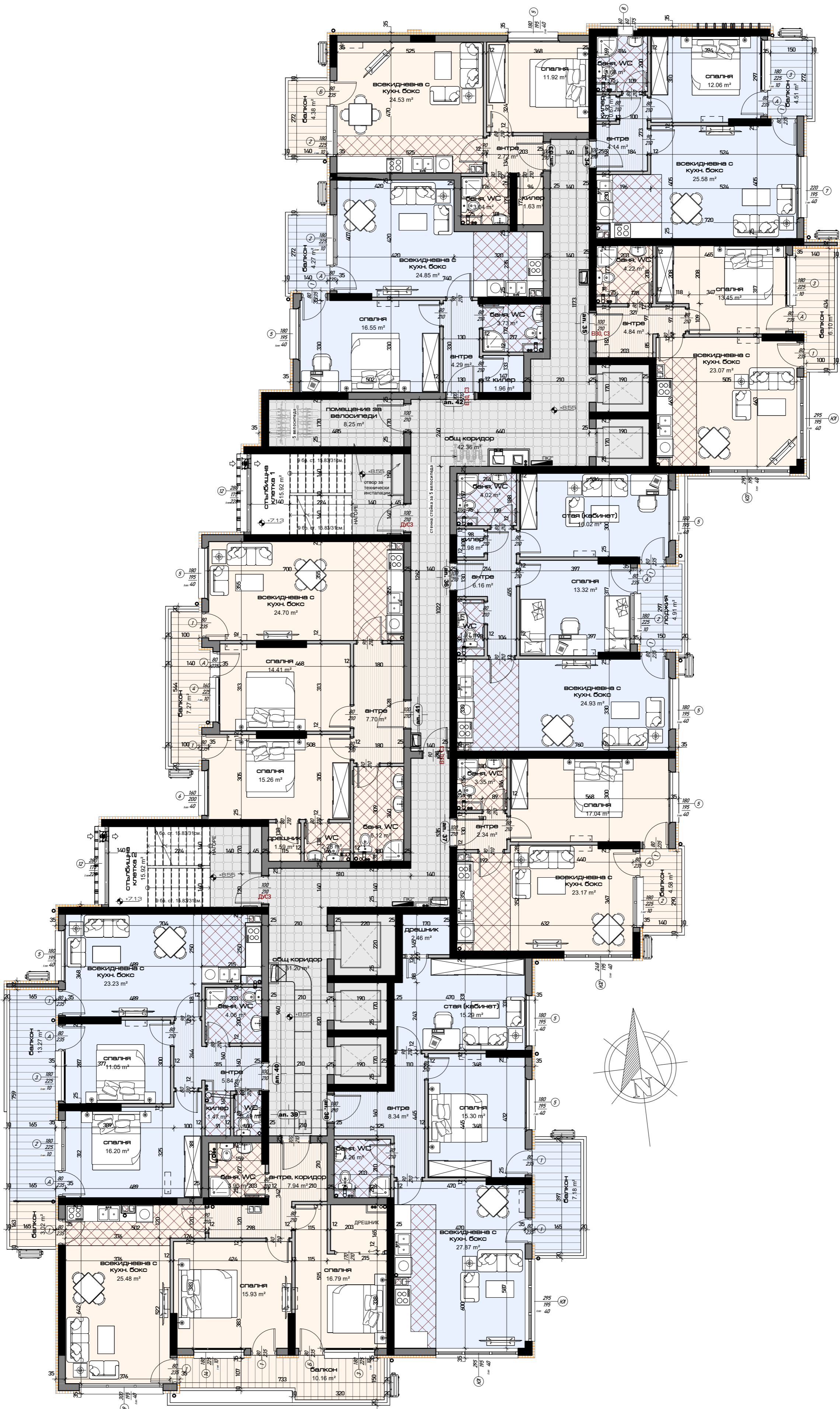
10 РАЗПРЕДЕЛЕНИЕ ЕТАЖ 5 (кт. +8.55м.) мащаб 1:100
