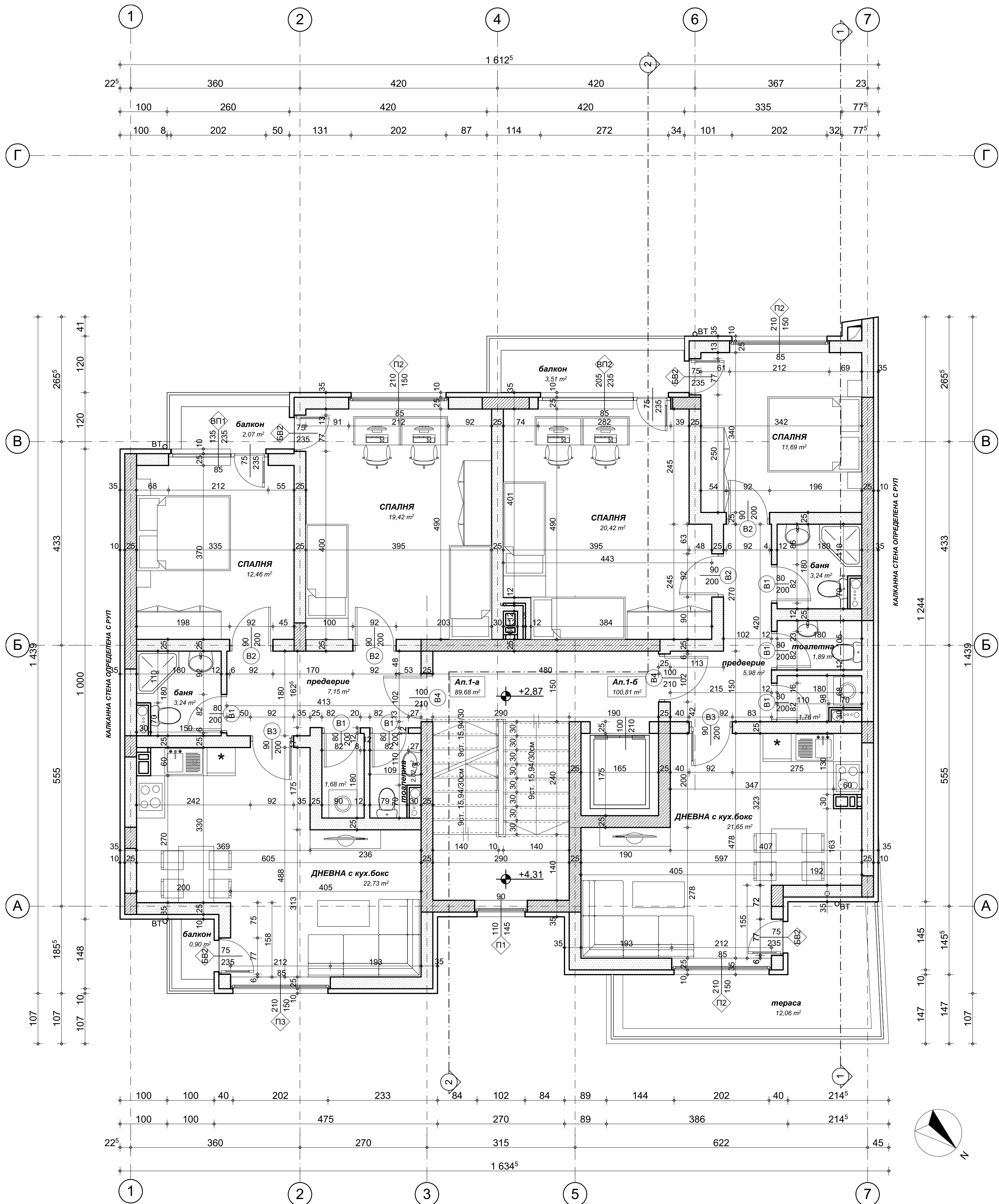
РАЗПРЕДЕЛЕНИЕ I ЖИЛИЩЕН ЕТАЖ M1:50
