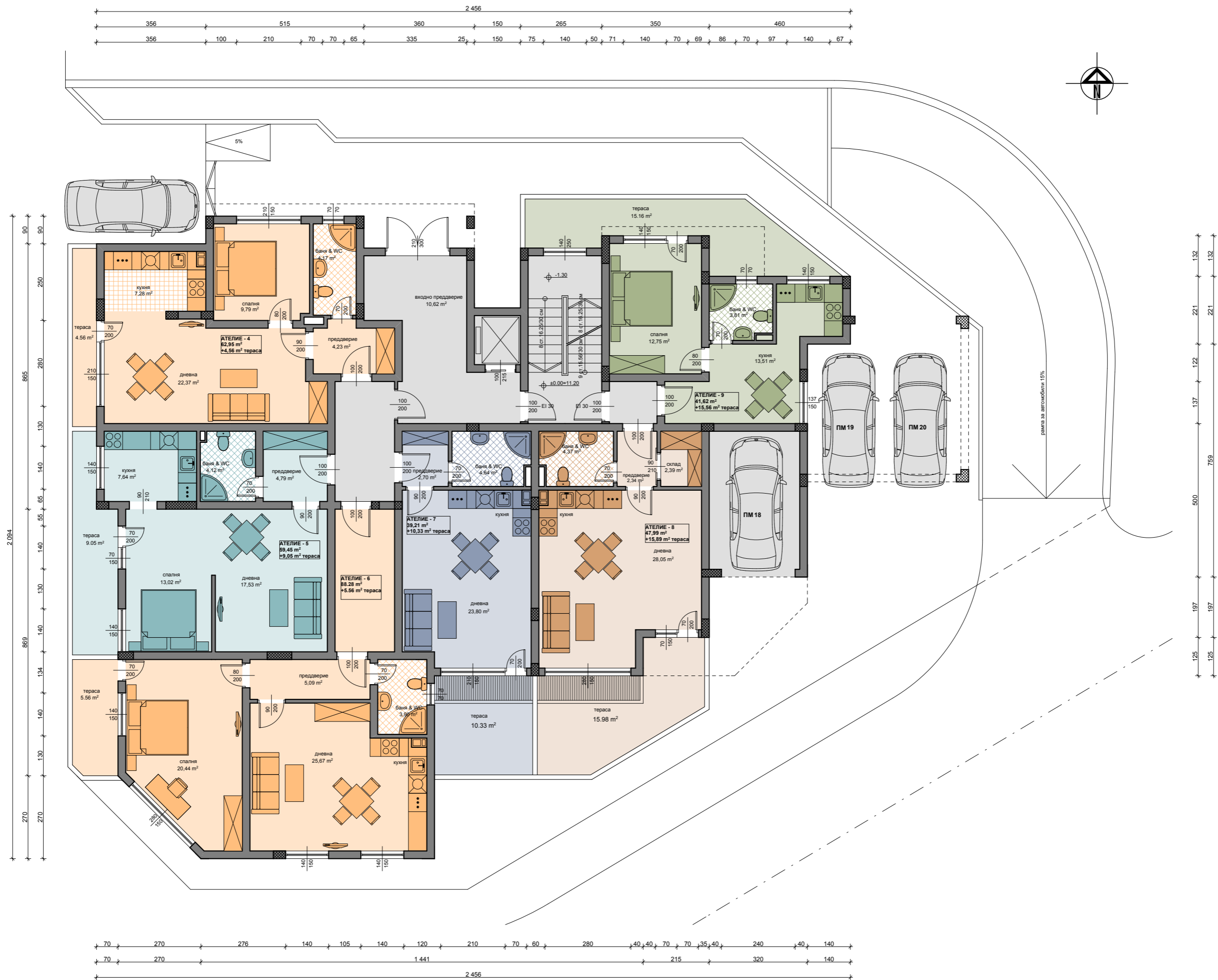
РАЗПРЕДЕЛЕНИЕ КОТА ±0.00
